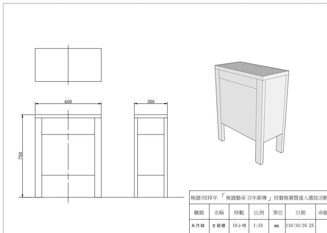
圖 1 家具規格示意圖
